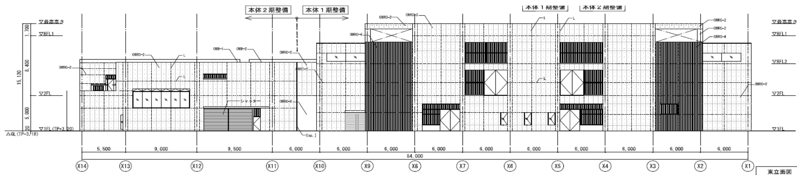
東側立面图
