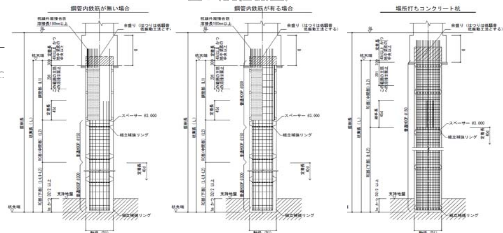
上部鋼管有・鋼管内配筋無し 上部鋼管有・鋼管内配筋有り RC杭(上部鋼管無し)
