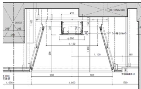
断面詳細図
