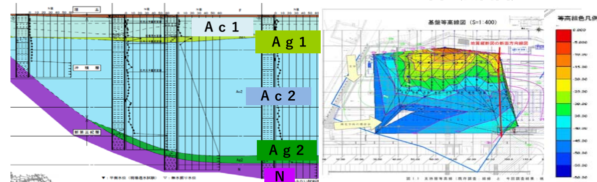
図3 (断面図)
