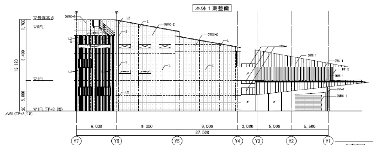
北側立面图
