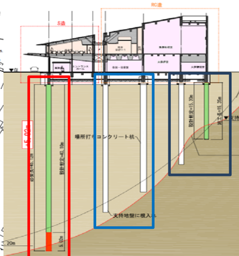
図3 (断面図)
