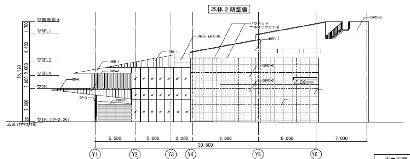
南側立面图
